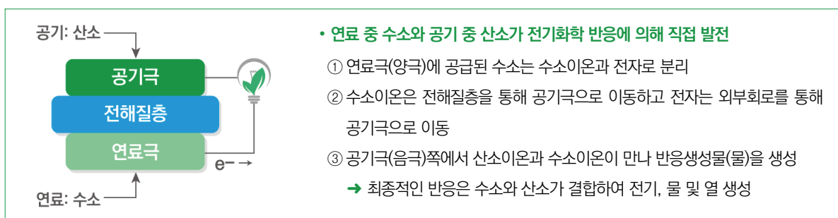
〈그림 43〉 연료전지 발전원리
