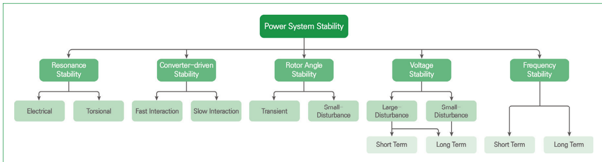
〈그림 30〉 IEEE 전력계통 안정도 분류
