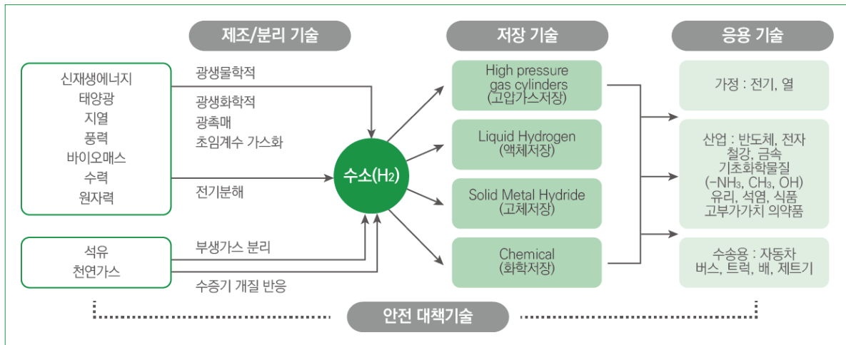
〈그림 42〉 수소에너지 시스템
