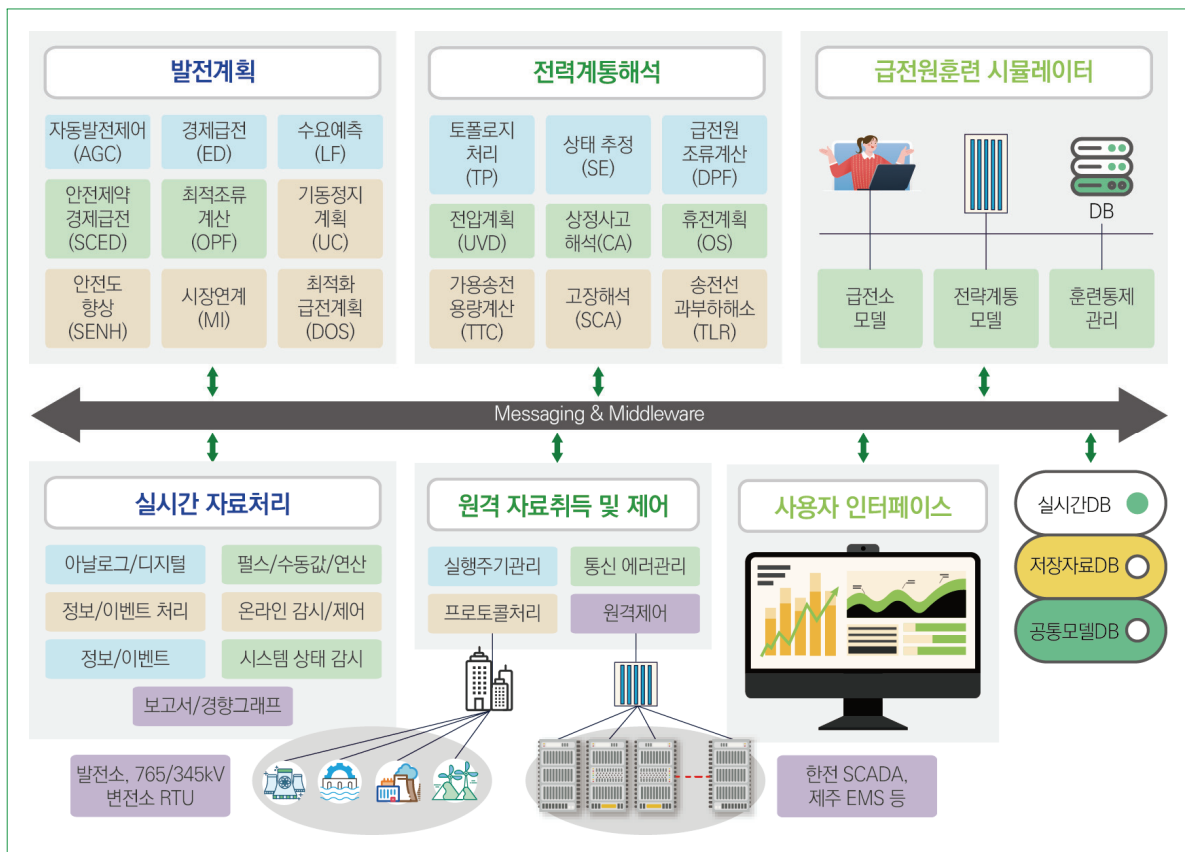
〈그림 29〉 한국형 EMS 기능 구성도
