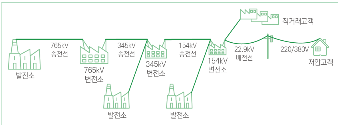
〈그림 28〉 전력계통 개념도
