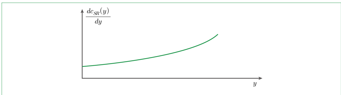
〈그림 19〉 전형적인 단기 한계비용함수
