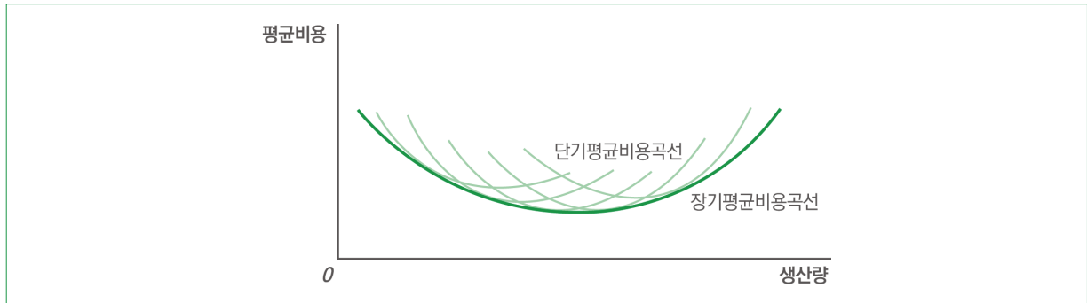
〈그림 1〉 단기평균비용곡선과 장기평균비용곡선
