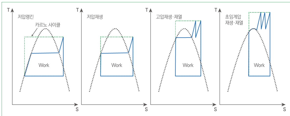
〈그림 16〉 각종 열 사이클의 열효율 비교
