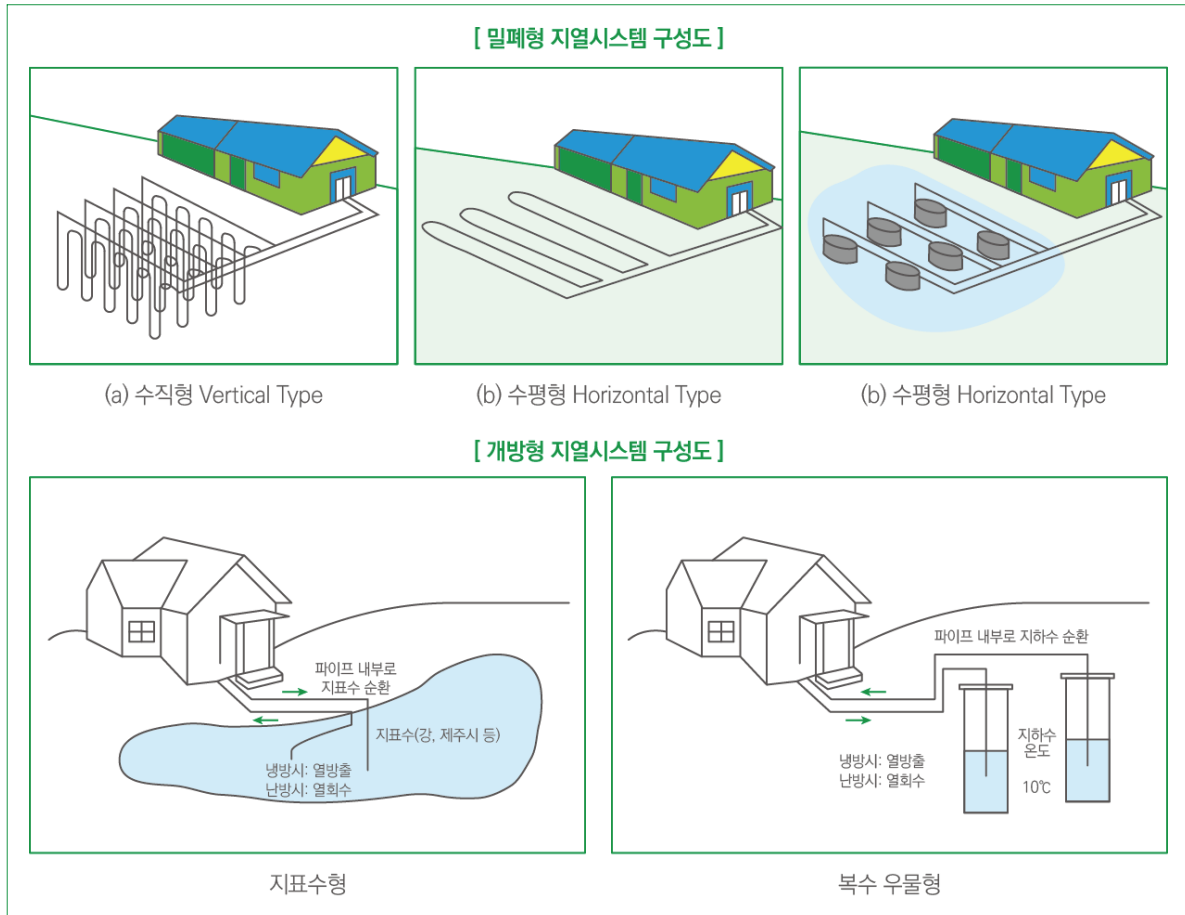
〈그림 49〉 지열 시스템 구성도
