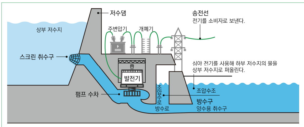
〈그림 47〉 수력발전시스템 모식도
