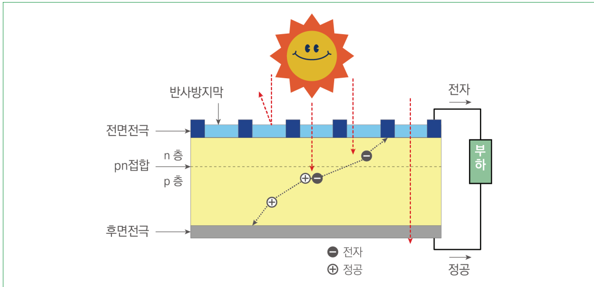
〈그림 11〉 태양전지 동작 원리
