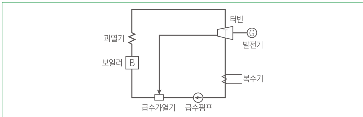
〈그림 15〉 열사이클의 블록선도
