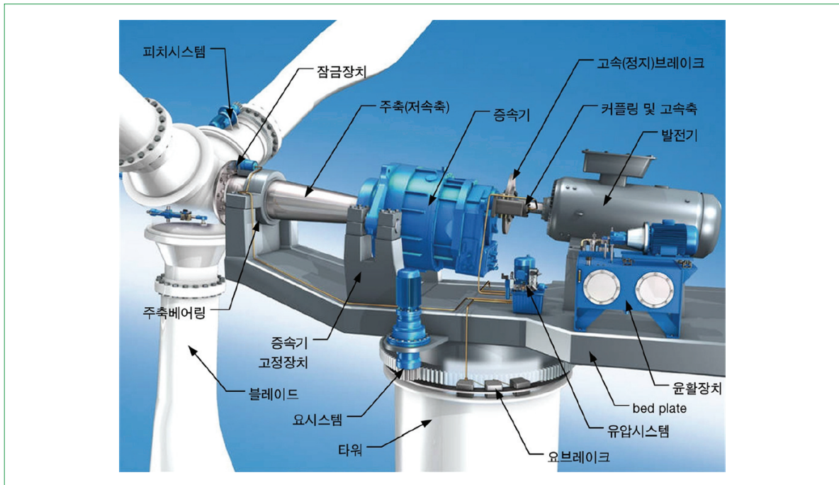
〈그림 46〉 풍력 발전기의 구조
