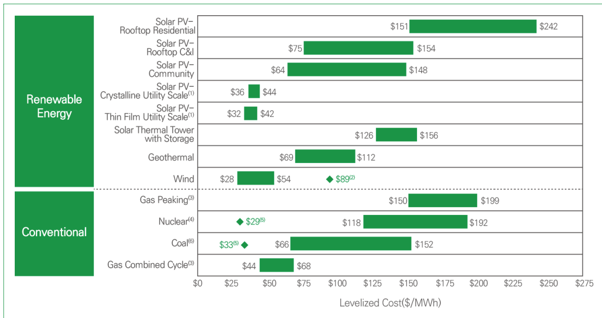
〈그림 26〉 2019년 글로벌 LCOE
