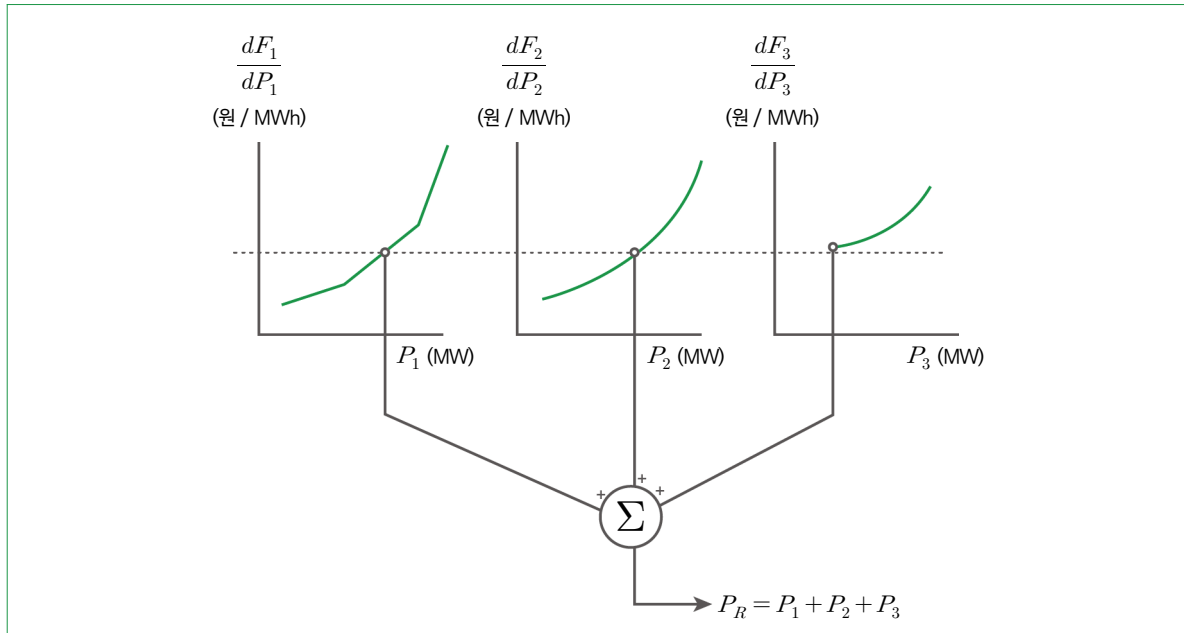
〈그림 20〉 경제급전의 도식해
