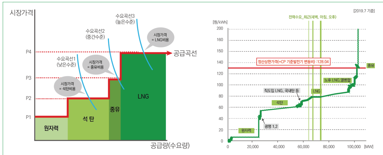
〈그림 5〉 전력시장 매시간 수요-공급곡선 형태 (이론 vs 실제)
