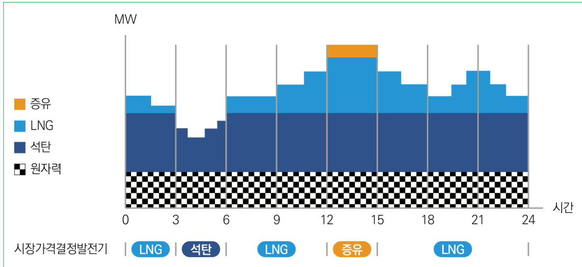
〈그림 38〉 계통한계가격의 결정 예시
