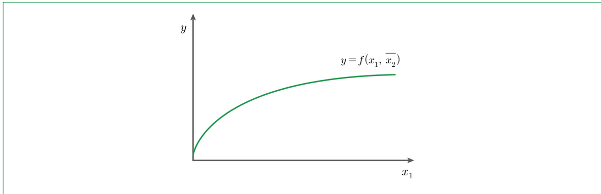
〈그림 17〉 전형적인 단기 생산함수
