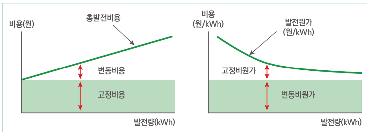
〈그림 40〉 발전량과 발전원가의 관계
