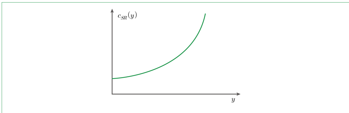
〈그림 18〉 전형적인 단기 비용함수
