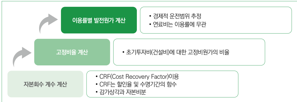
〈그림 27〉 LCOE 산정절차
