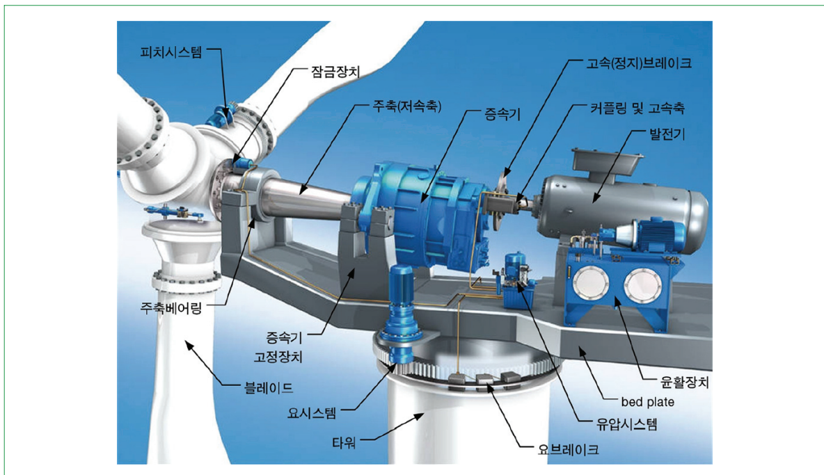
〈그림 12〉 풍력발전기 구조
