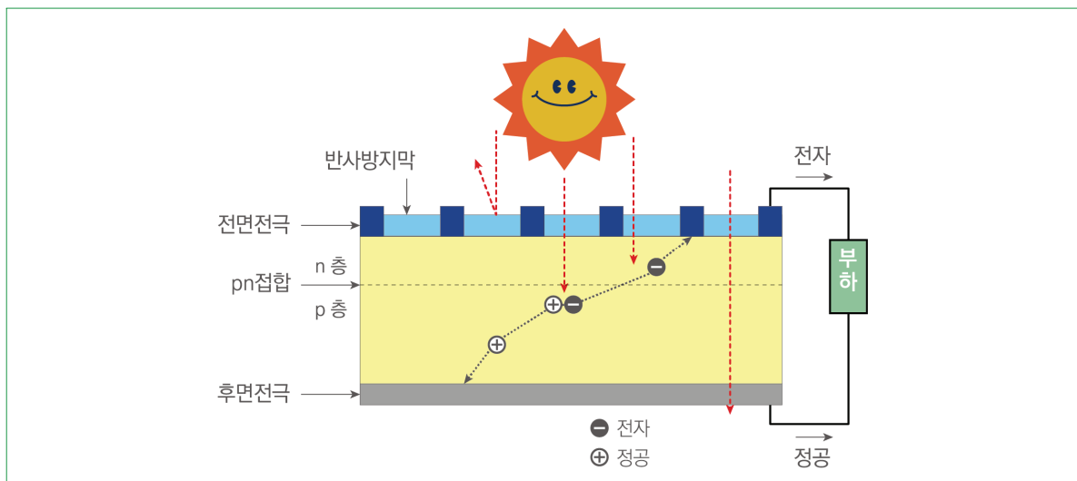
〈그림 45〉 태양전지 동작 원리
